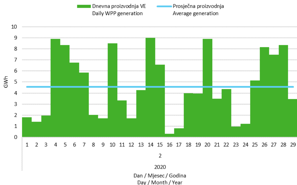
Slika 5 Dnevna proizvodnja svih vjetroelektrana u veljači 2020. godine Figure 5 Daily generation of all wind power plants in February 2020
