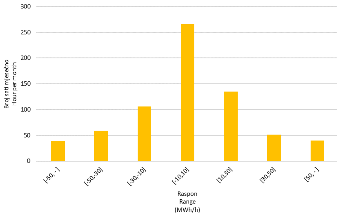
Slika 10 Statistička raspodjela satnih promjena proizvodnje VE u veljači 2020. godine
