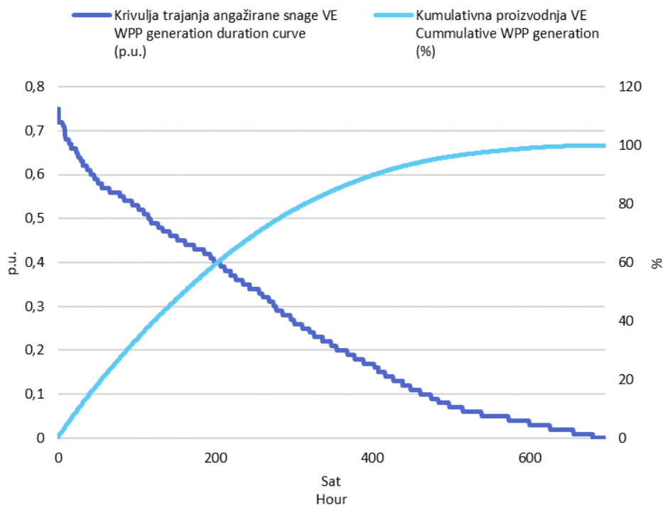
Slika 3 Krivulja trajanja angažirane snage svih VE i kumulativna proizvodnja VE u veljači 2020. godine u jediničnim vrijednostima
