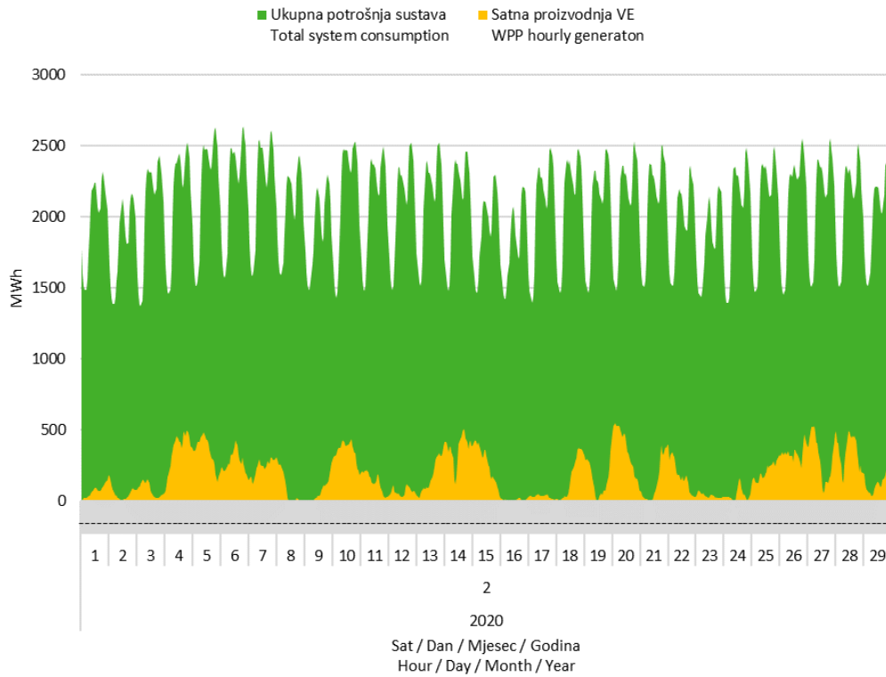
Slika 7 Usporedba satnog dijagrama opterećenja sustava i proizvodnje vjetroelektrana u veljači 2020. godine
