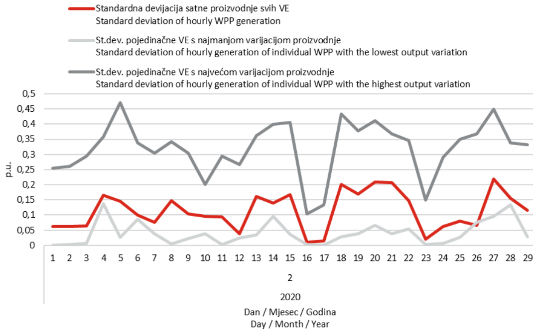
Slika 4 Standardna devijacija satne proizvodnje vjetroelektrana u jediničnim vrijednostima Figure 4 Standard deviation of hourly generation of all wind power plants in per unit
