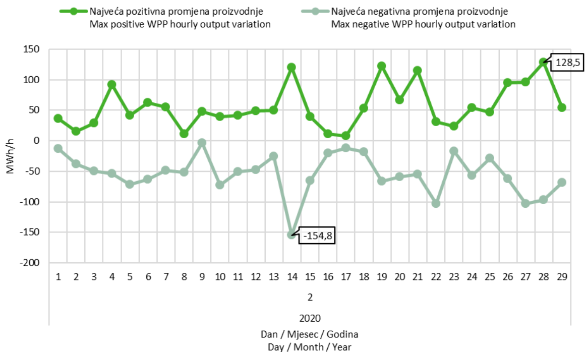
Slika 9 Maksimalna pozitivna i maksimalna negativna promjena satne proizvodnje VE u veljači 2020. godine
