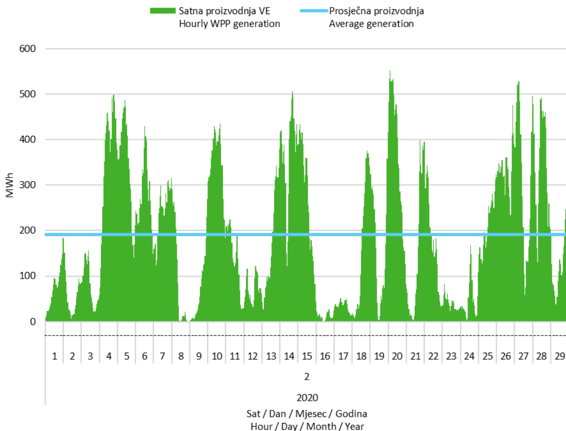
Slika 2 Satna proizvodnja svih vjetroelektrana u veljači 2020. godine Figure 2 Hourly generation of all wind power plants in February 2020
