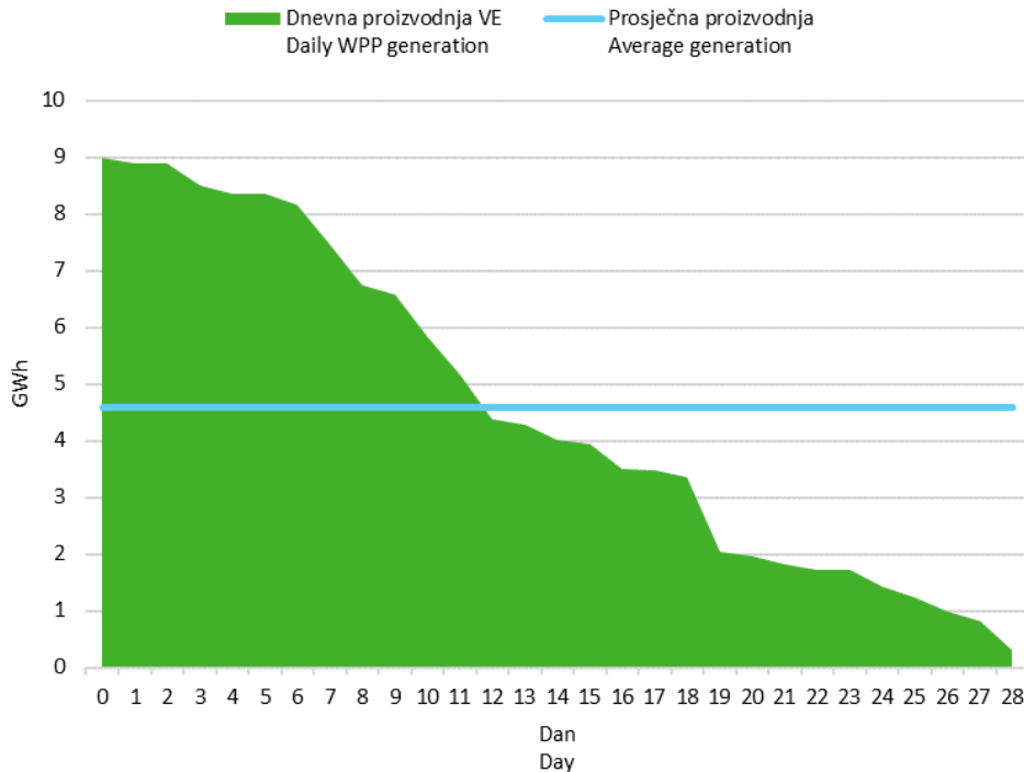
Slika 6 Krivulja trajanja dnevne proizvodnje vjetroelektrana u veljači 2020. godine
