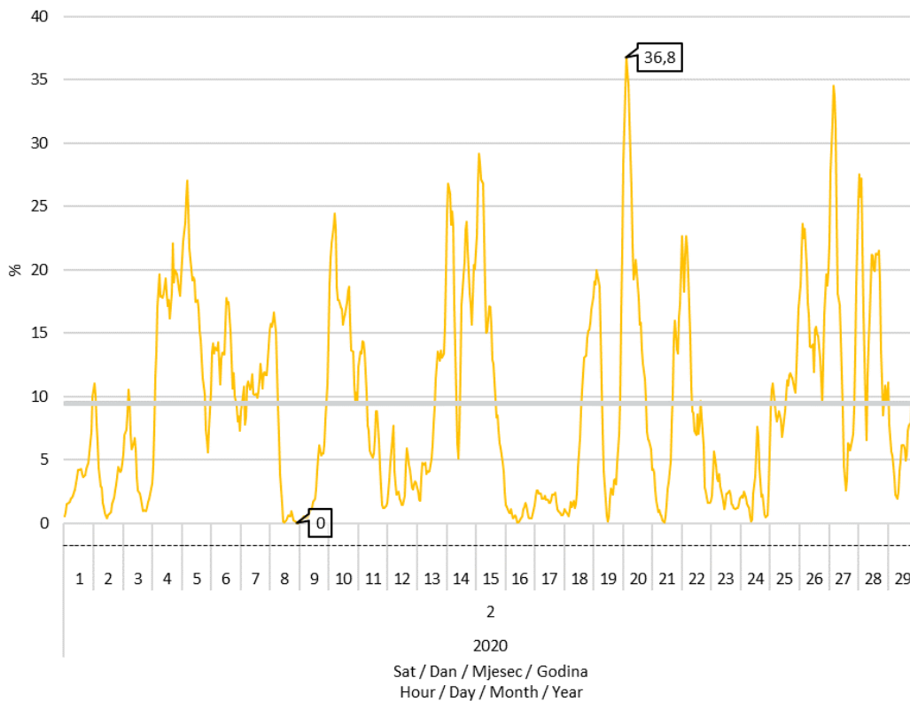
Slika 8 Udio proizvodnje vjetroelektrana u pokrivanju satnog opterećenja elektroenergetskog sustava u veljači 2020. godine
